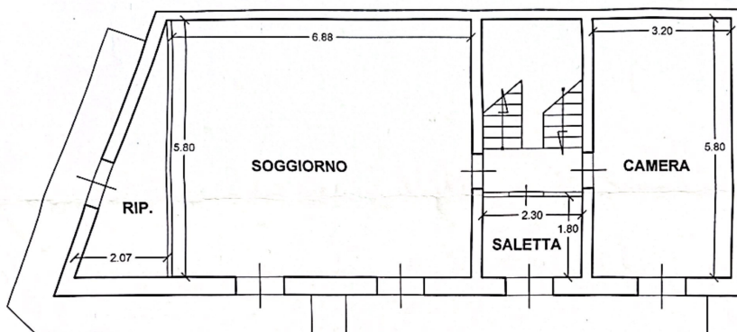
PIANTA PIANO PRIMO H= 4.35 ml
