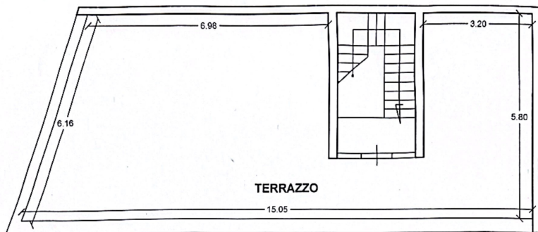
PIANTA PIANO DI COPERTURA H= 2.30 ml SCALA 1/1
